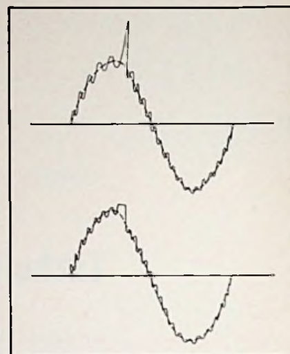
Bild 2. Einer sinusförmigen Schwingung mit niedriger Frequenz ist die Pilotfrequenz von 19 kHz überlagert.
