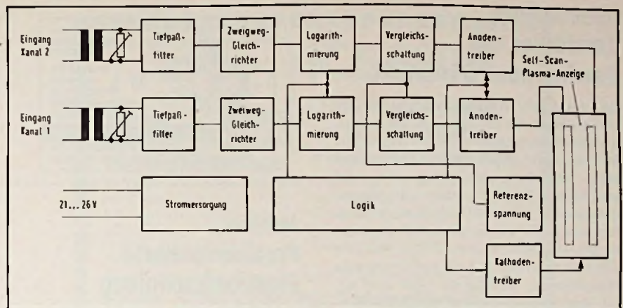
Blockschaltung des vollelektronischen Stereo-Aussteerungs-Instruments
