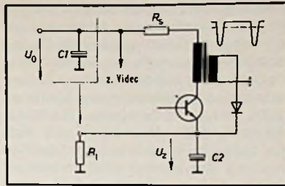
Bild 1. Prinzip der kontrollierten Zwischenspannung C 1 – Ausgangskondensator im Netzteil (rd. 50 \mu\text{F} ) C 2 – Ladekondensator der kontrollierten Zwischenspannung U_z R s – Schutzwiderstand der Zeilenendstufe (rd. 100 \Omega ) R 1 – Belastung der kontrollierten Zwischenspannung durch die nachfolgenden Stufen
