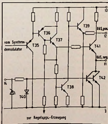
Bild 4. Videoverstärker
