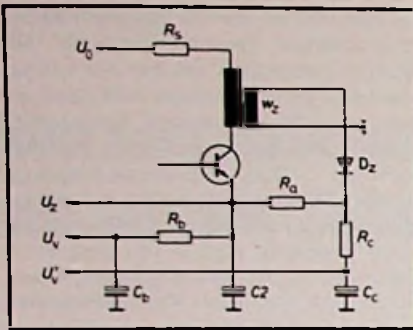
Bild 3. Gewinnung der Hilfsspannung U' zur Definition der Vertikalampplitude U_v – Betriebsspannung der Vertikalablenkschaltung
